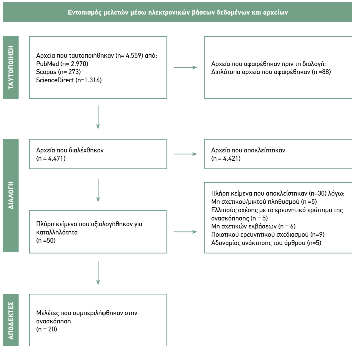
Σχήμα 1 - Διάγραμμα Ροής PRISMA
